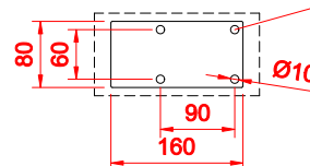
ROZSTAW OTWORÓW MONTAŻOWYCH
